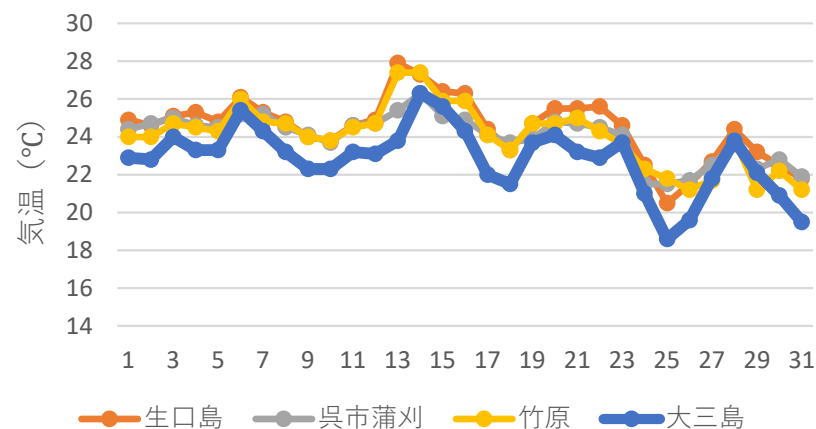
2019年8月 日最低気温
