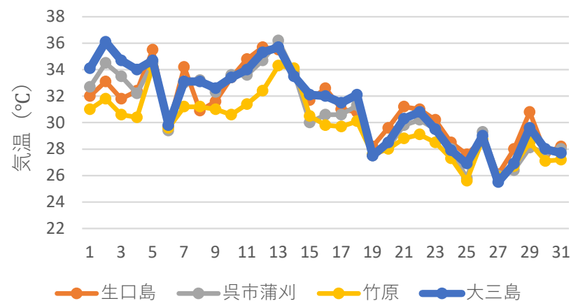
2019年8月 日最高気温
