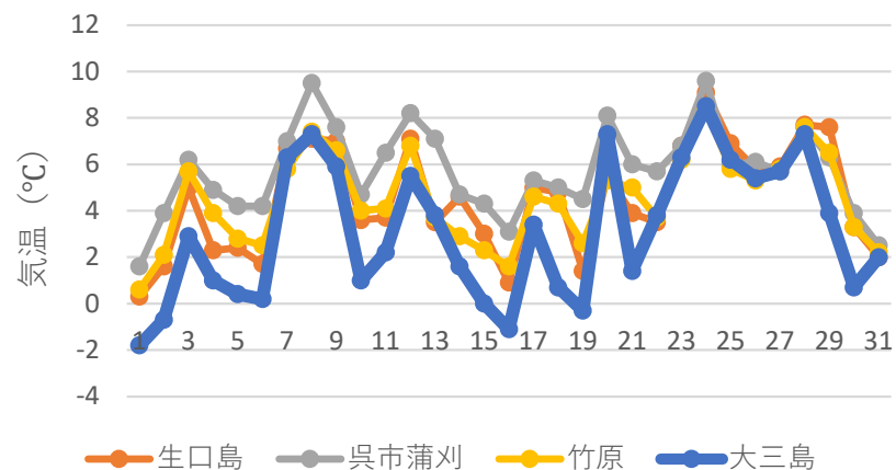
2020年1月 日最低気温
